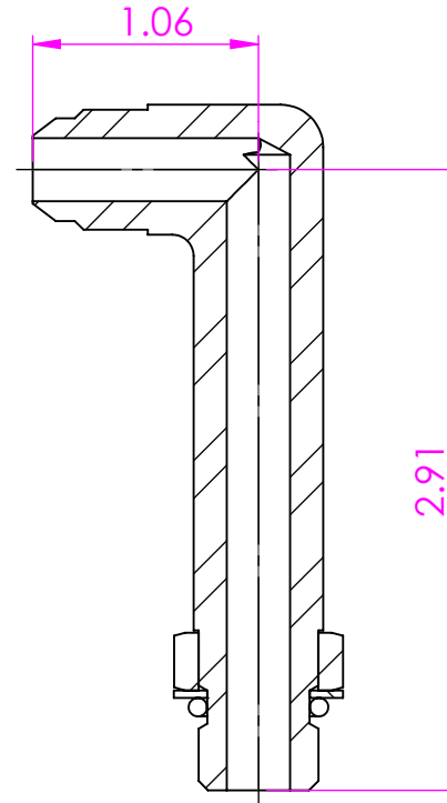
SECTION A-A
